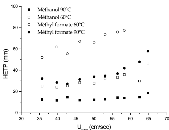
Figure V.8.: Dépendance de l'efficacité de la colonne MXT U en fonction de la vitesse du gaz vecteur pour le méthanol et le méthyl formate. Conditions opératoires : T=60^\circ\text{C} et 90^\circ\text{C} , p_o=20 kPa.
