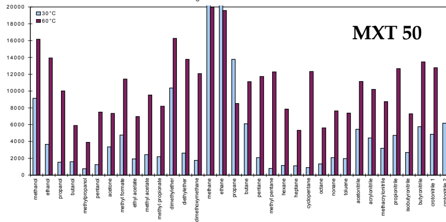
Figure IV.7. : Evolution de l'efficacité des colonnes à film liquide étudiées en fonction de la température.
