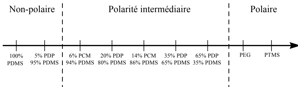
Figure III.7. : Echelle de polarité (non linéaire) des phases stationnaires liquides les plus employées.
