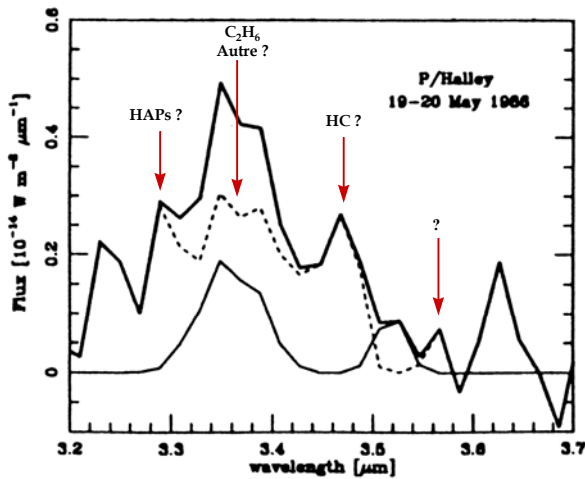
Figure I.8. : Spectre de la coma de P/Halley entre 3,2 et 3,7 μm (ligne épaisse) et spectre résiduel (pointillés) après soustraction de la contribution du méthanol (ligne fine) (adapté de (Bockelée-Morvan et al., 1995)).
