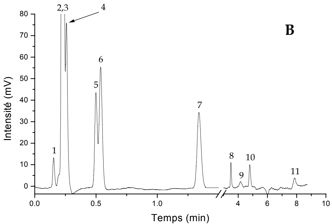
Figure V.13. : Séparation chromatographique d'un mélange des gaz ciblés par la colonne Carbobond. Conditions opératoires : p_i=150 kPa, p_o=1 kPa, (A) T=30^\circ\text{C} , (B) T=60^\circ\text{C} . Pics : 1=Ne, 2= \text{N}_2 , 3=Ar, 4=CO, 5= \text{CH}_4 , 6=Kr, 7= \text{CO}_2 , 8= \text{C}_2\text{H}_2 , 9=Xe, 10= \text{C}_2\text{H}_4 , 11= \text{C}_2\text{H}_6 .
