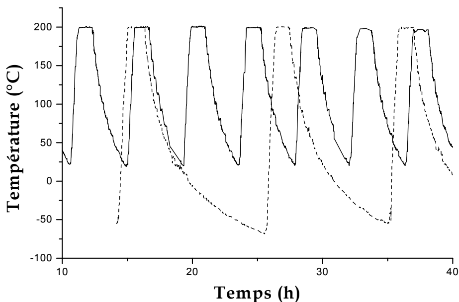
Figure V.1. : Cycles de températures enregistrés durant les tests de cycles thermiques.
